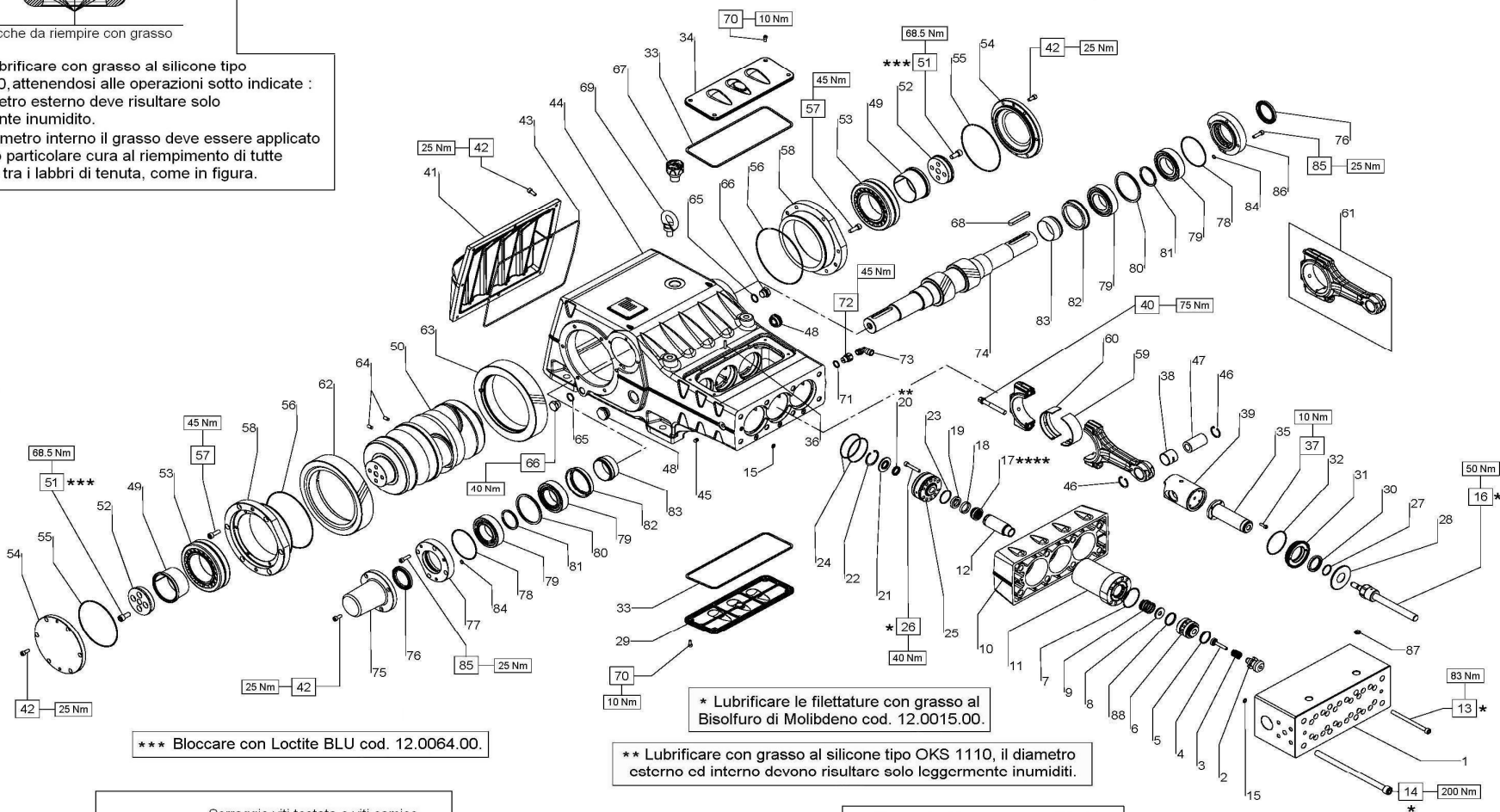
Serraggio viti supporto guarnizioni pos. 26
